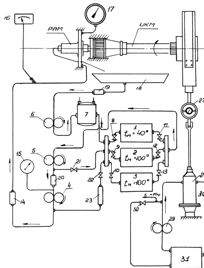
Рис.1 Существующая гидравлическая схема испытательного комплекса для обкатки, тарировки и испытания ИКМ. 1.,2.,3-маслобаки.4-помпа ИКМ.5-подкачивающая помпа., 6-откачивающая помпа.7-радиатор. 8-,9,10,11,12,13 -краны.14-фильтр,15,17-манометр,16-термометр, 18-поддон, 19,20-фильтры,21-кран регулятора подкачки,22-кран расходомера,23-жиклер,27-динамометр, 28-цилиндр,29-помпа нагрузки,30-кран регулировки нагрузки,31-маслобак
